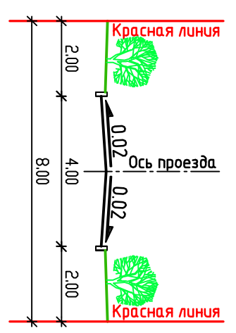
Поперечный профиль ул. Школьная
