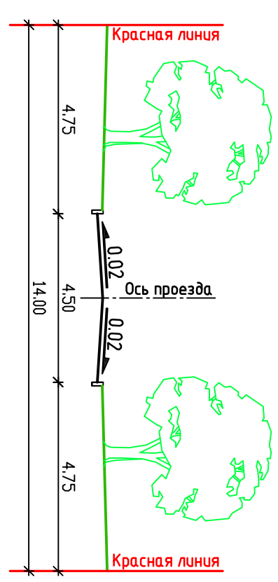
Поперечный профиль 2-20 Коммунального пер.
