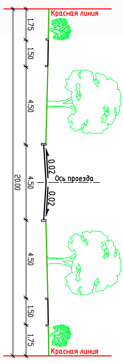
Поперечный профиль ул. Труда и ул. Коммунальная
